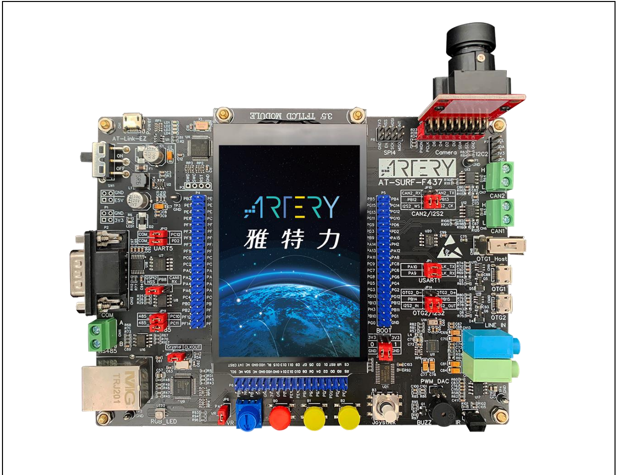
图 1. AT-START-F437 V1.0 开发板
